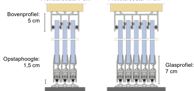
3-sporig Profielbreedte: 7 cm
